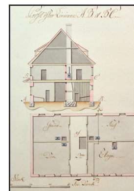
Tegning av indre vakt: I 1775 ble det fastsatt at det skulle oppføres en andre etasje på den eksisterende bygningen. (EA-5930 Riksarkivets kart- og tegningssamling, IB 12).
